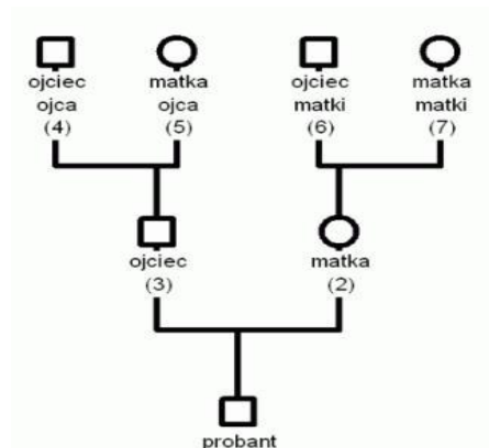
Ryc. 2. Tablica ascendentów
